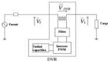
Figura.2. Esquema típico de un DVR
