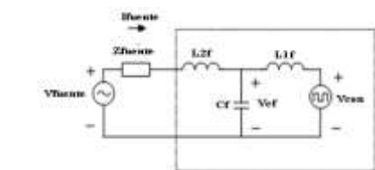
Figura.3. Filtro LCL aplicado a un convertidor paralelo
