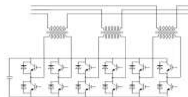
Figura.5. Convertidor de puente completo con transformador en Y/Y
