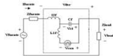
Figura.4. Filtro LCL aplicado a un convertidor serie
