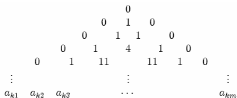
Fig. 2 Triángulo numérico generado por los coeficientes a_{km}
