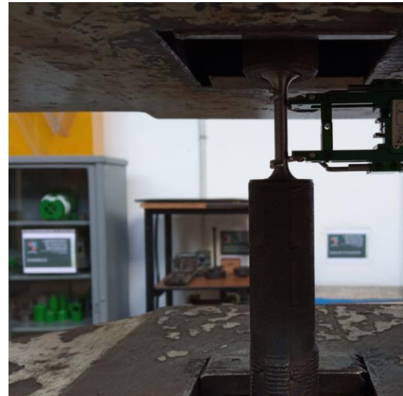
Fig. 10. Realización del ensayo de tracción.
