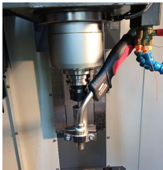
Fig. 1. Sistema de sujeción de la antorcha.
