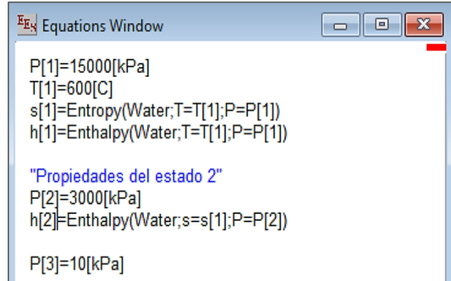
Fig. 4. Programación en EES de las propiedades termo físicas para los estados 1 y 2. Fuente: Esta investigación, software E.E.S.
