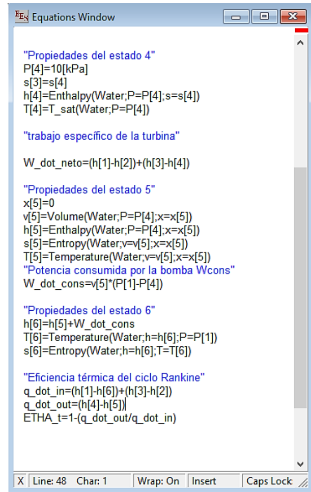
Fig. 9. programación del ciclo Rankine ideal con recalentamiento en EES fuente: esta investigación.
