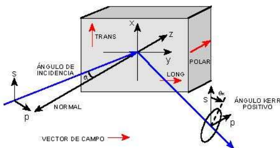
Figura 1. Geometría de la polarización para una muestra magnetizada.
