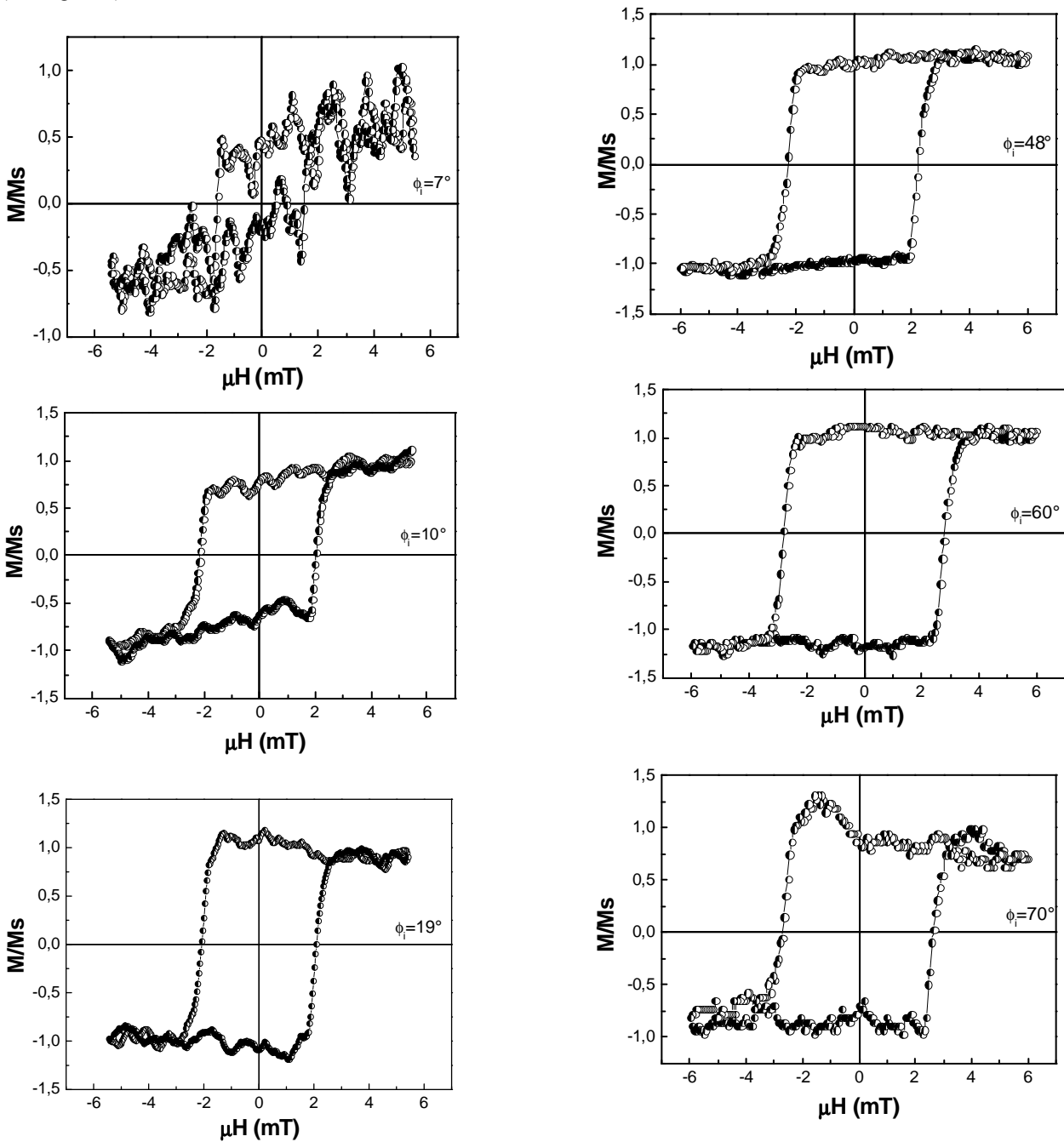
Figura 2. Ciclos de histéresis para diferentes ángulos de incidencia del haz lumínico en el magnetómetro Kerr.
