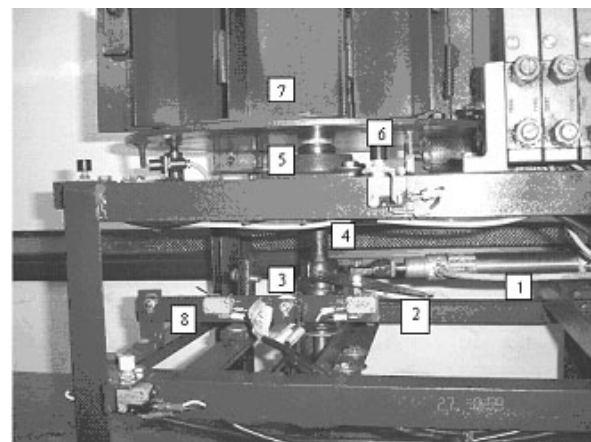
Figura 5. Mecanismo para el giro de la mesa
