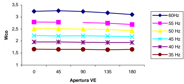
Figura 4. Variación del trabajo del compresor en función de la frecuencia del compresor y la apertura de la válvula de expansión.
