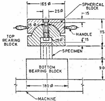
Figura 4. Apoyo hemisférico de la máquina universal.
