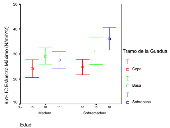
Figura No.10 edad y tramo de la guadua VS esfuerzo máximo de compresión.
