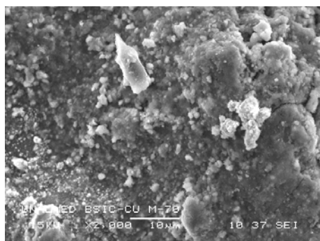
Figura 7. \beta -SiC modificado con Cu
