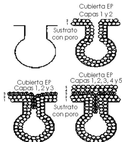
Figura 6. Mecanismo del recubrimiento por monocapas evidenciado en el proceso EP
