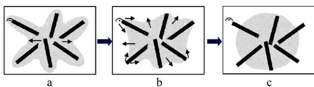
Figura 5. Modelo de Kim y Lee: (a) Composite (b) Transformación \text{CuO} ( \text{Cu}_2\text{O} ), aumento de volumen e incremento del contacto, formación de cuellos en el punto de contacto, (c) Geometría generada para disminuir la energía superficial, partículas aglomeradas
