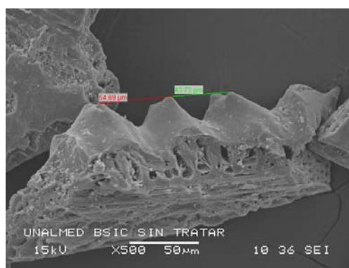
Figura 3. Micrografía SEM de \beta -SiC obtenido por pirólisis de CA
