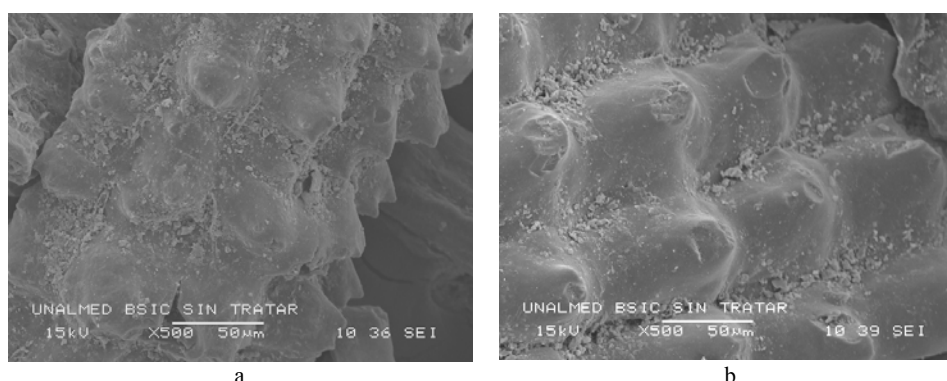
Figura 2. Micrografía SEM de \beta -SiC obtenido por pirólisis de CA
