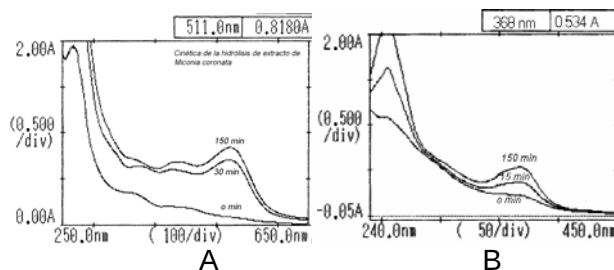
Figura 4. Espectros de los hidrolizados de taninos condensados (A) y taninos hidrolizables (B) a diferentes tiempos de reacción.
