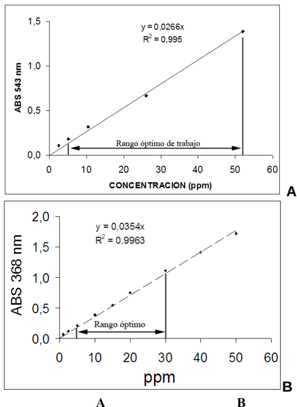
Figura 5. Curva de calibración de malvidin para estimación de taninos condensados (A) y de ácido elágico para estimación de taninos hidrolizables (B)
