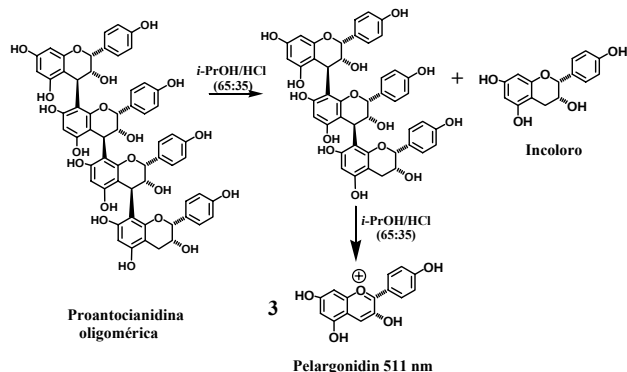
Figura 2. Hidrólisis ácida de un tetrámero de pelargonidin.
