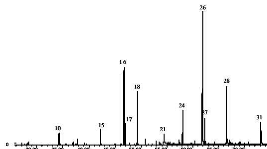
Figura 1. Perfil cromatográfico del absoluto de las flores de Posoqueria latifolia : 10-Eugenol, 15-metoxyeugenol, 16-N.I. 17-benzoato de bencilo, 18-salicilato de bencilo, 21- ácido linolénico, 24-Tricosano, 26-<1>-Pentacosano, 27-Pentacosano, 28-HC, 31-HC.
