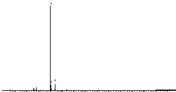
Figura 2. Compuestos mayoritarios de la fragancia de las flores de Posoqueria latifolia : 4- cis -3-Acetato de hexenilo, 5-acetato de hexilo, 6- a-cis -ocimeno
