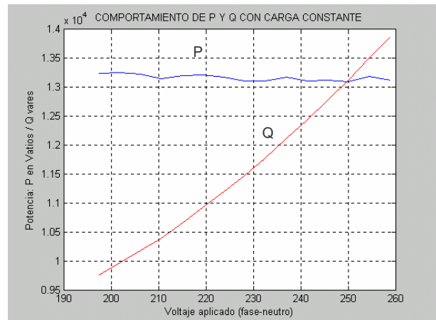
Figura 4. Motor de 20 Hp con variación de voltaje desde 0,9V_n hasta 1,18V_n y torque de carga constante de 80N-m
