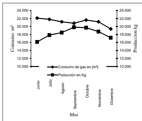
Figura 1. Consumo de gas y producción antes y después de implementación de la mejora.
