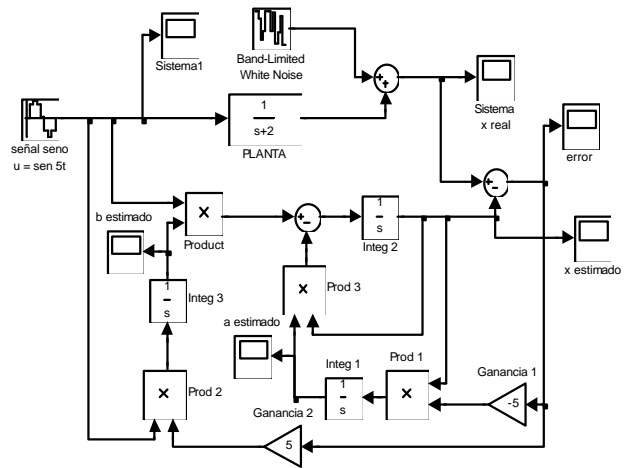
Figura 4. Diagrama de simulación para modelo paralelo.
