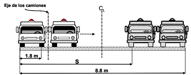
Figura 14. Esquema de los vehículos moviéndose juntos desde
