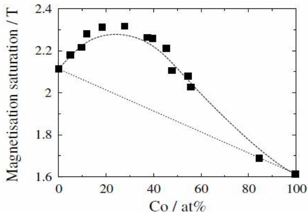
Figura8: Magnetización de saturación del sistema FeCo en función del contenido de cobalto (Tomado de T. Sourmail [20]).
